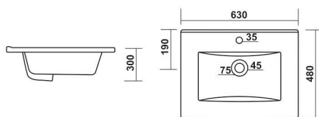
101-AQUA TOP COUNTER
