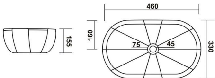
7016-SLEEK L 460 W 330 H 155mm
